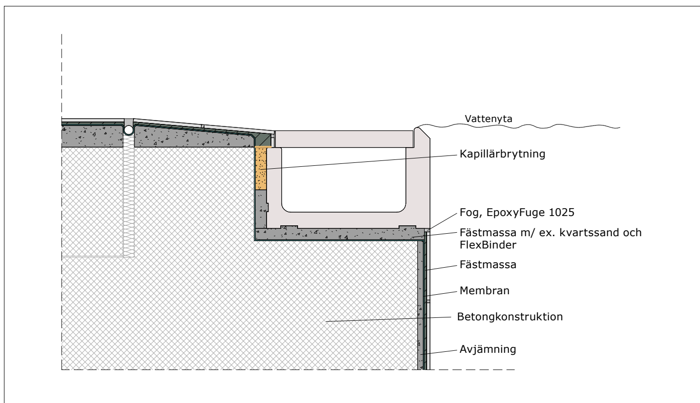
Exempel på montering av skvalpränna
